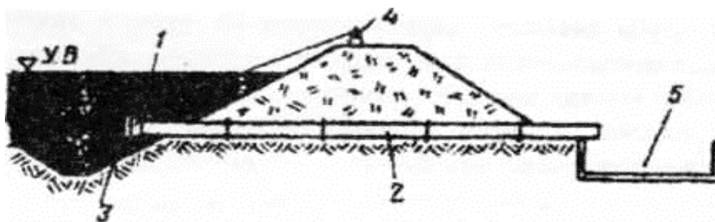
Донный водоспуск упрощенного типа: 1 - оголовок с решетками, 2 - водопроводная часть (лежак), 3 - клапанный затвор. 4 - лебедка, 5 - уловитель личинок;
