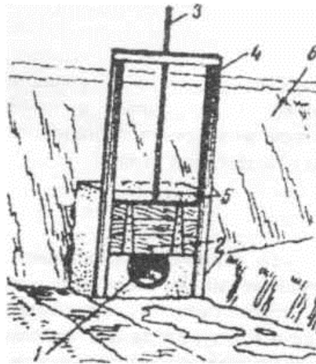
Донный водоспуск без стока: 1 - отверстие труб, 2 - щит, 3 - стержень для подъема и спуска щита, 4 - железные швеллеры - пазы для движения щита, 5 - бетонный оголовок. 6 – низовой откос дамбы
